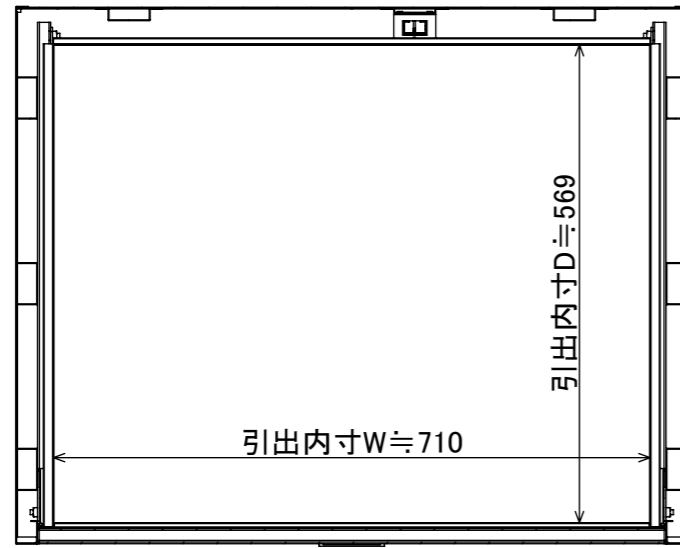
断面図 A-A
