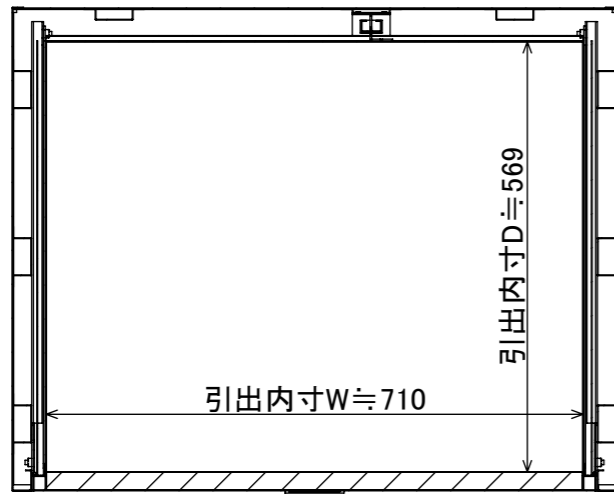
断面図 A-A
