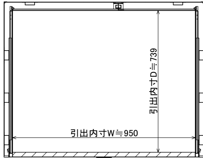
断面図 A-A
