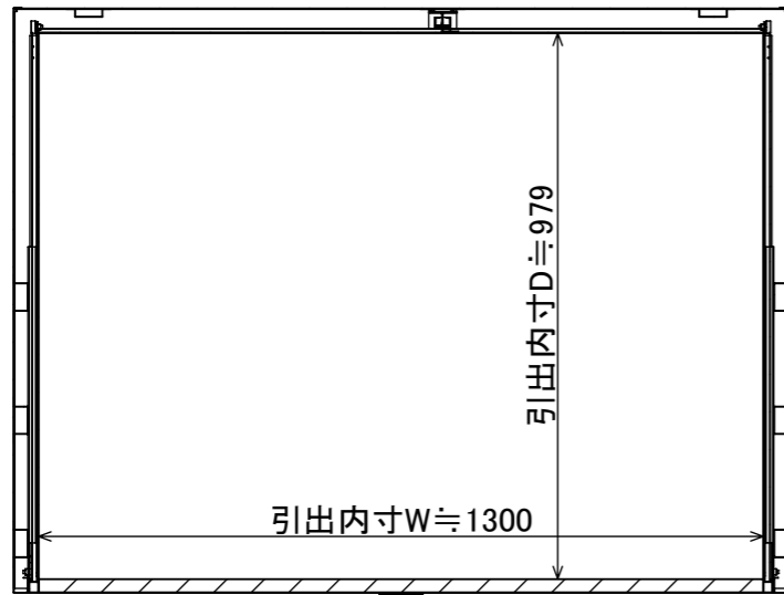
断面図 A-A
