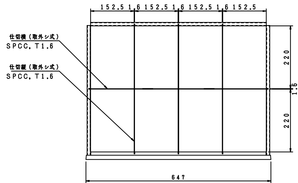
間仕切寸法
