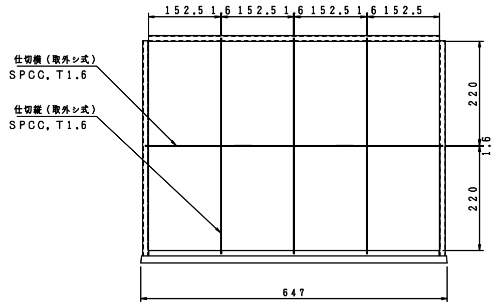
間仕切寸法
