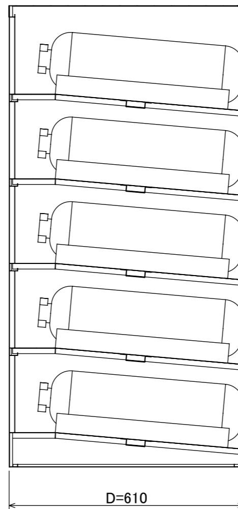
断面図 A-A
