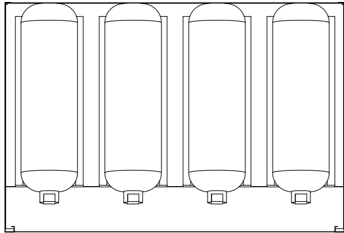
断面図 B-B
