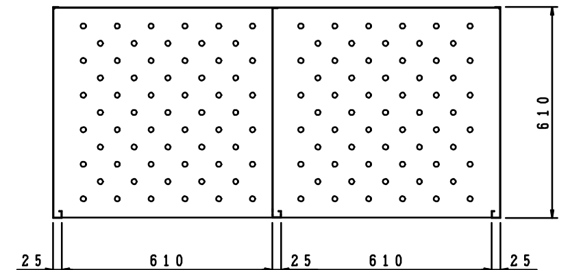
下段収納庫本体横断面
