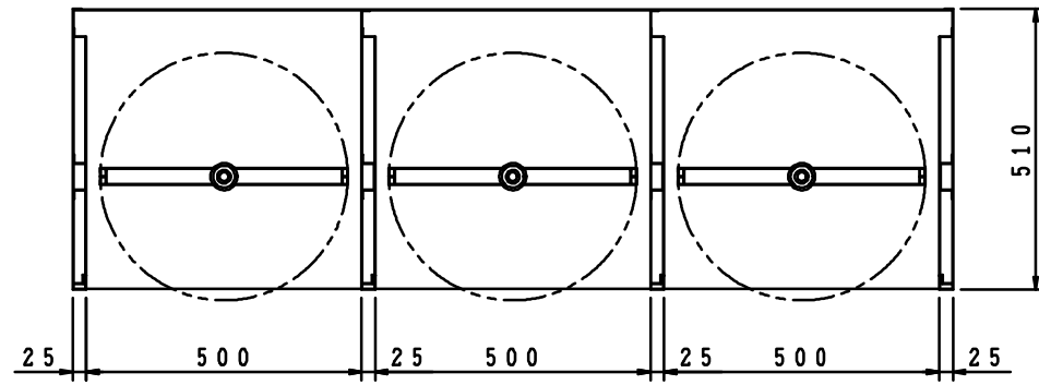
防火衣収納庫本体横断面
