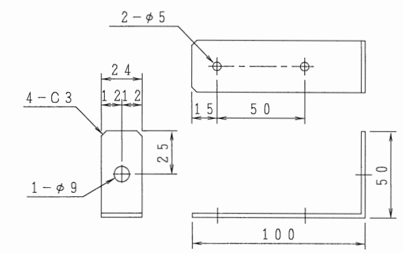
壁固定金具 S=1/3
