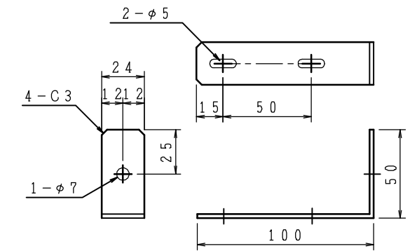
壁固定金具 S=1/3
