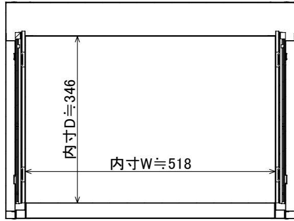
断面図 A-A
