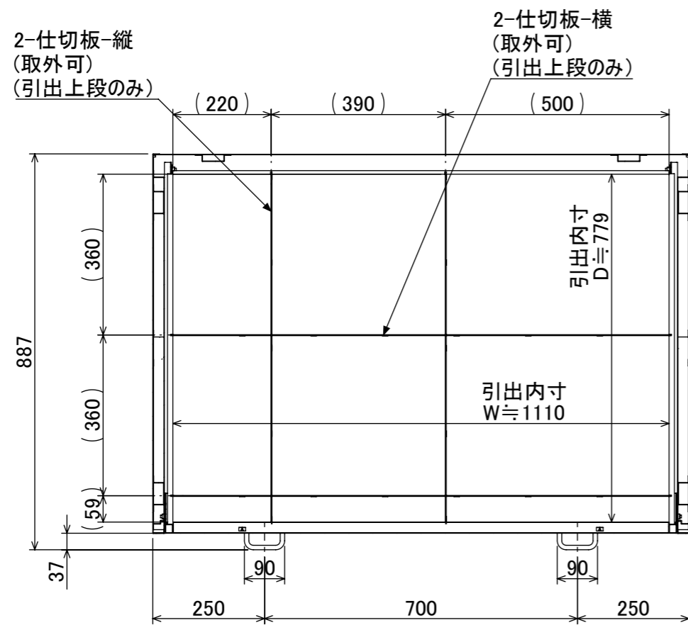
断面図 A-A
