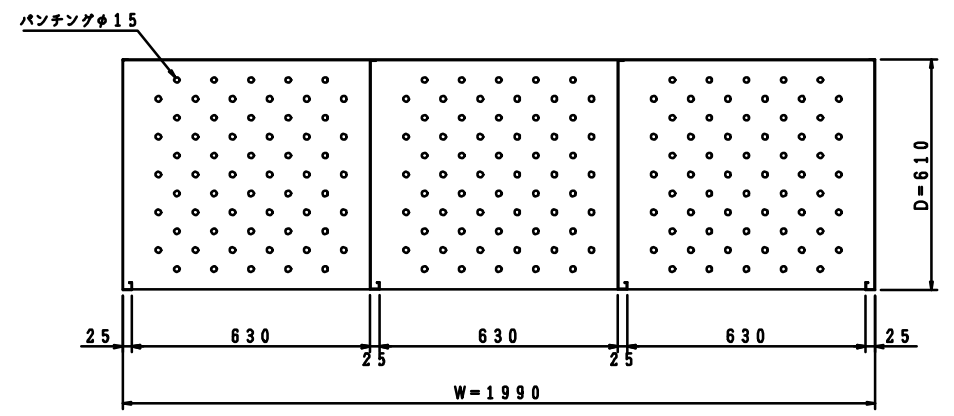
下段収納庫横断面
