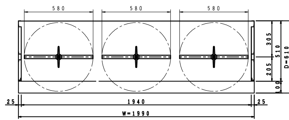
防火衣収納庫横断面
