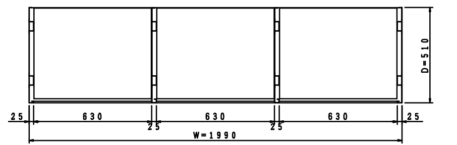
上段収納庫横断面
