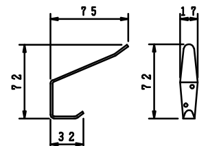
ステンレス帽子掛 (S=1/5) SUS304-ヘアライン
